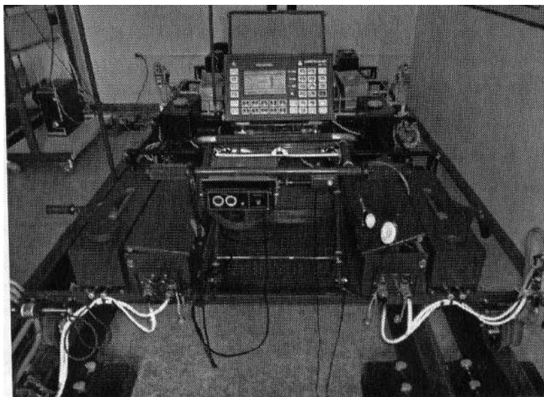
Дефектоскоп «Авикон-01»
