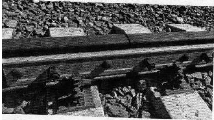
Рис. 13. Стыковое скрепление
