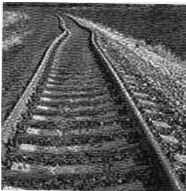
Рис. 40. Выброс железнодорожного пути
