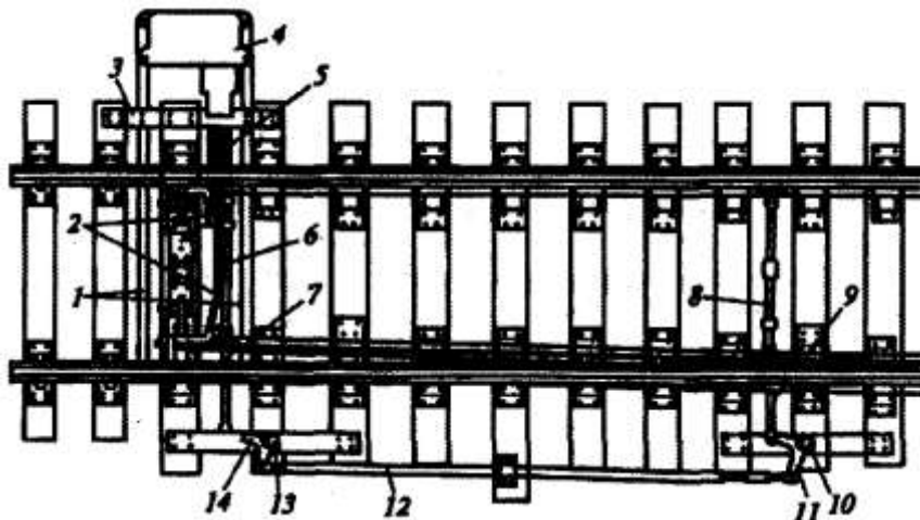
Переводное устройство и гарнитура на стрелках с гибкими острьяками
