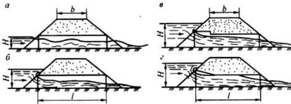
Рис. 45. Схемы водопрпускных труб
