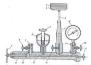
Рис. 17.10. Малометр с пневматической пружиной
