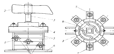
Рис. 6.2. Пакетный выключатель. 1 — стальная шина; 2 — рукоятка; 3 — вилки для переключения подвижных дисков; 4 — корпус; 5 — пакеты; 6 — основание; 7 — винтовые контакты для подключения проводов; 8 — подвижные диски с контактами
