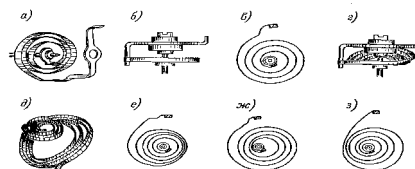
Рис. 3.10. Различные виды повреждения спиральных пружинок: а-в – правильное положение пружинок; д – скручивание; е – изгиб в плоскости лужины; г, ж, з – неправильная привалка пружинок
