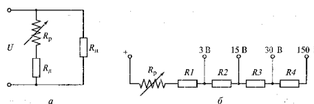
Рис. 3.20. Схемы включения добавочного резистора:
