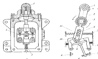
Рис. 6.4. Подвижные контакты переключателя (а) и выключателя (б) типов
