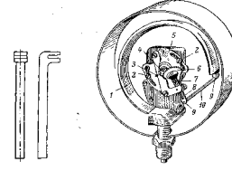
Рис. 17.8. Малометр с пневматической пружиной
