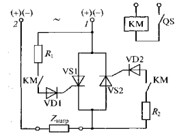
Рис. 6.26. Принципиальная электрическая схема тиристорного контактора
