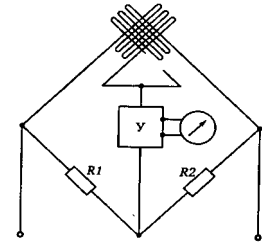
Рис. 3.6. Мостовая схема включения тензодатчика
