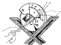
Рис. 3.9. Определение противодействующего момента спиральной пружины прибора
