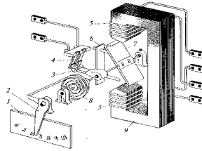
Рис. 6.27. Реле максимального тока серии РТ
