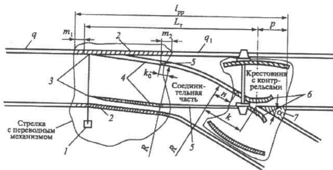
Рис. 38. Конструкция одиночного обыкновенного стрелочного перевода
