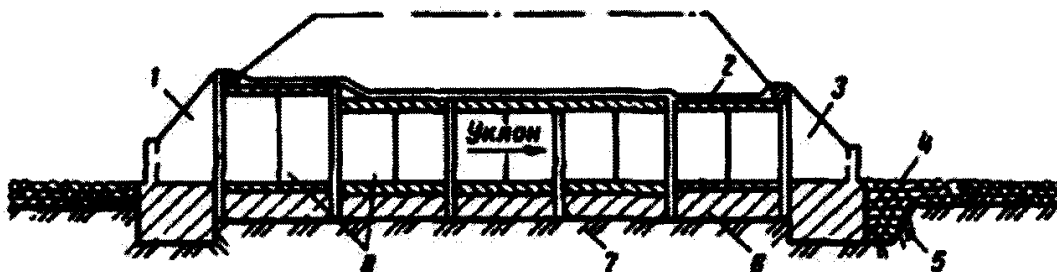
Рис. 41. Искусственное сооружение
