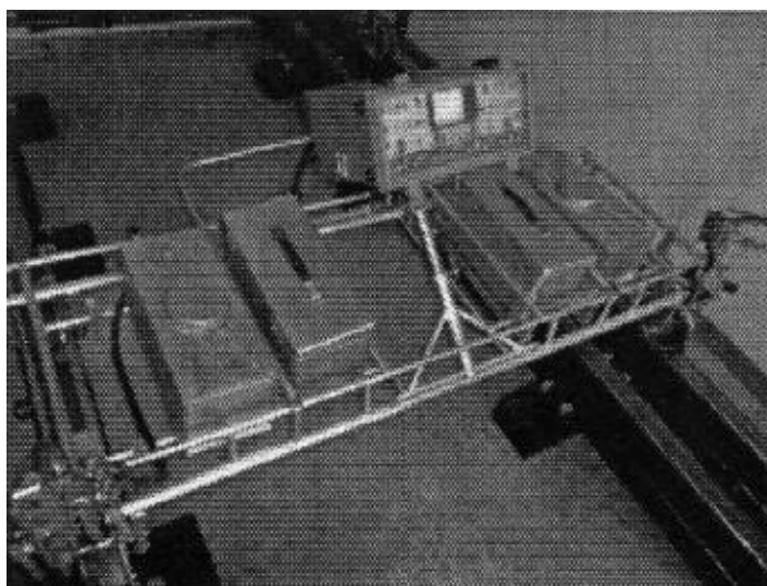
Ультразвуковой дефектоскоп «Поиск-10», лаборатория «Неразрушающий контроль рельсов»
