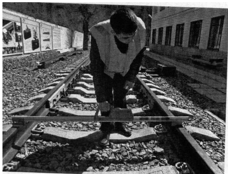
Рис. 14. Измерение шаблоном ширины рельсовой колеи
