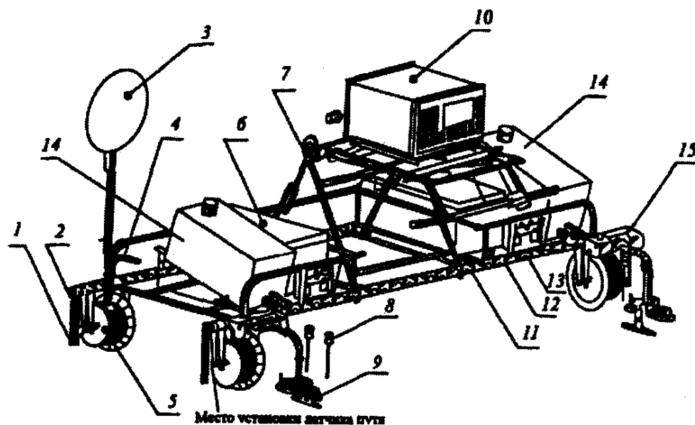
Схема дефектоскопа
