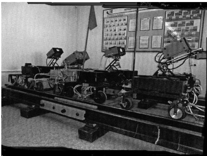
Образцы дефектоскопов
