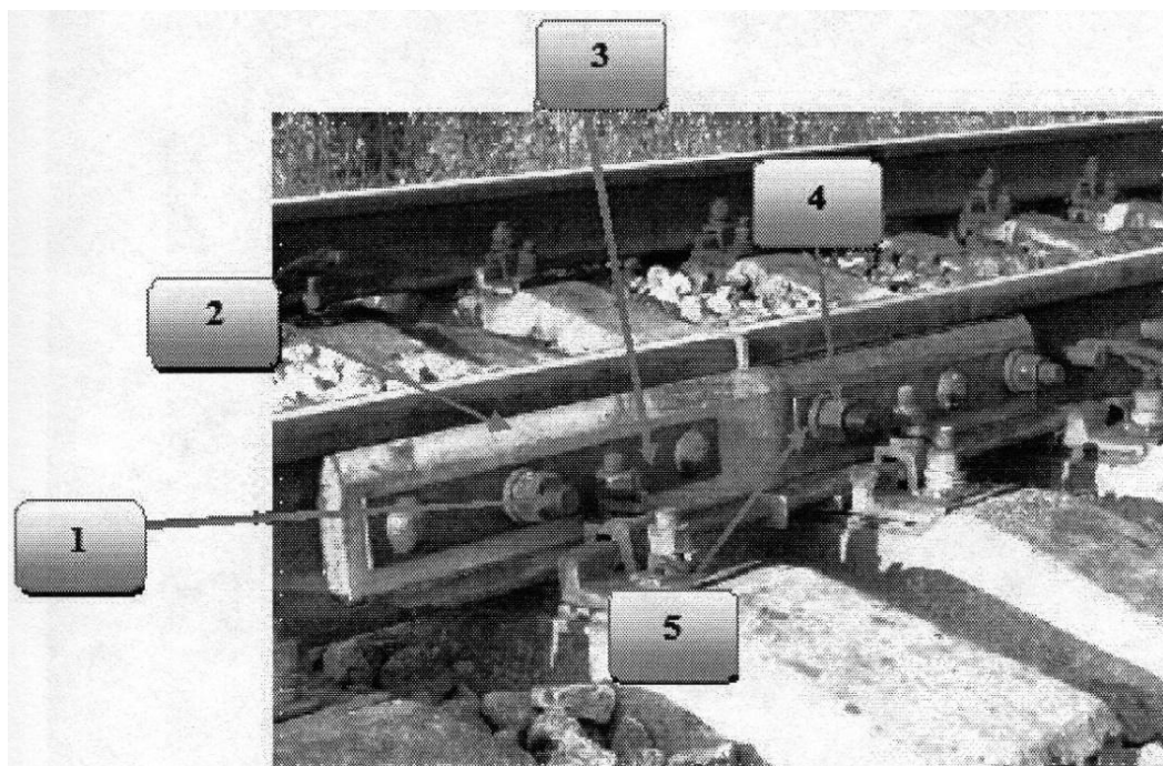
Рис. 3. Стык изолирующий
