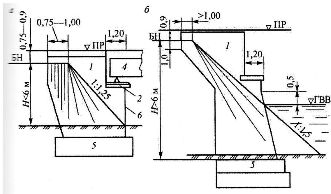
Рис. 47. Виды опор
