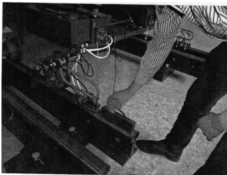
Ультразвуковой дефектоскоп «Авикон-01», лаборатория «Неразрушающий контроль рельсов»
