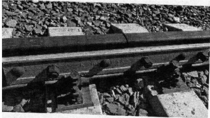
Рис. 13. Стыковое крепление
