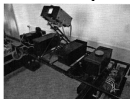
Ультразвуковой дефектоскоп «РДМ-2», лаборатория «Неразрушающий контроль рельсов»
