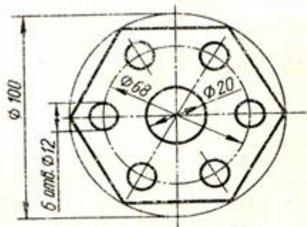
Решетка
